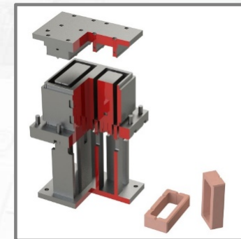
Оснастка для выпуска облицовочных строительных элементов методом полусухого прессования
